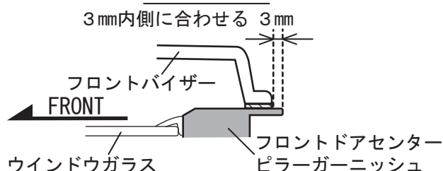
断面 d-d'
