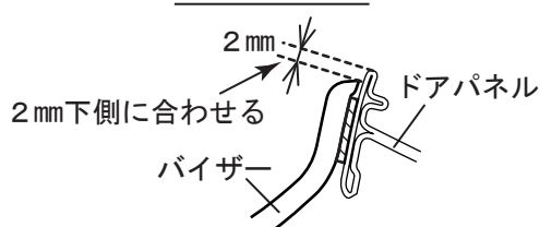
断面 d-d'
