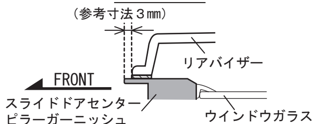
断面 g-g'
