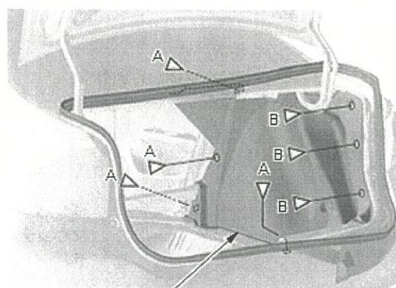
トランク リヤ サイド ライニング
