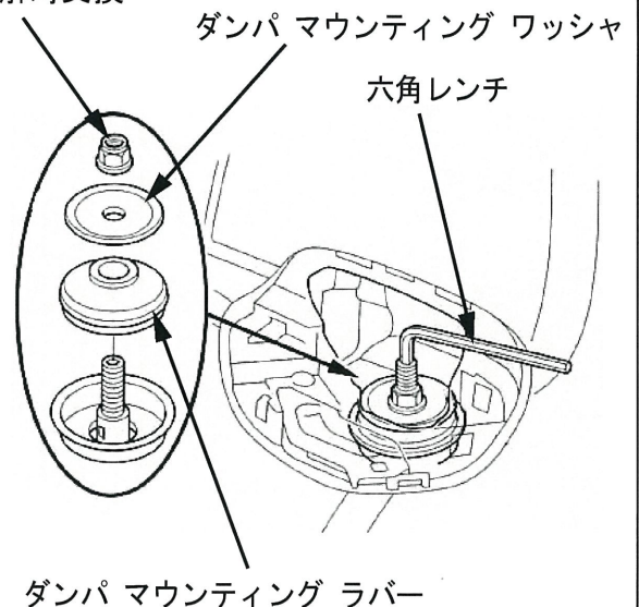
ダンパ上部取付けナット
