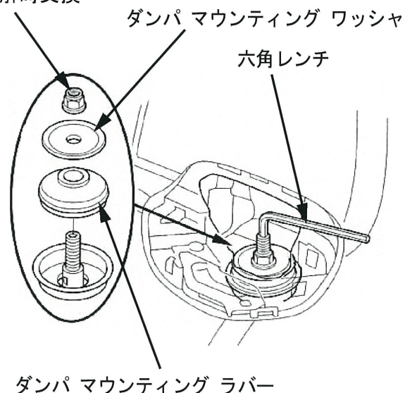
ダンパ上部取付けナット
