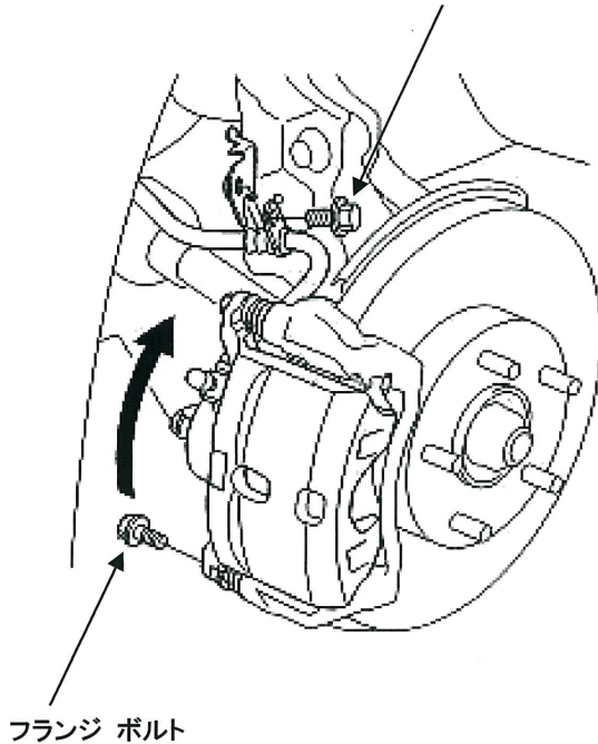
ブレーキ ホース クランプ ボルト
