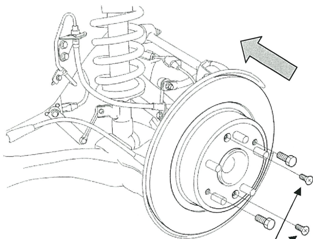
フラット スクリュ 6×1.0mm 9.8N・m(1.0kgf・m)
