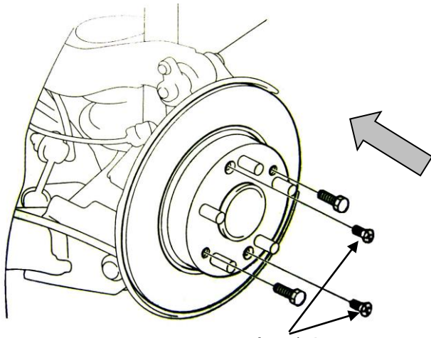
フラット スクリュー 6×1.0mm 9.8N・m(1.0kgf・m)
