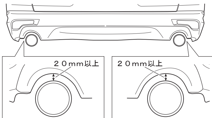
〔後面視〕
